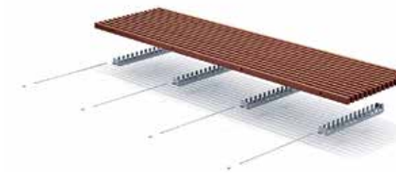
Peigne breveté Streetlock® en acier inoxydable avec tige et écrous de serrage antivol.
